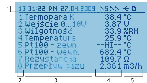
Rys.12.2. Wygląd ekranu listy pomiarów w trybie TYLKO TEKST (dla ilości kanałów większej od 8 dane prezentowane są w dwóch kolumnach, bez nazw, podgląd nazw dostępny jest w kolejnych widokach)
