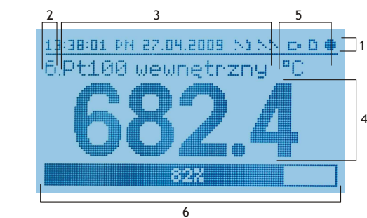
Rys.12.4. Wygląd ekranu pojedynczego pomiaru w trybie DUŻE ZNAKI
