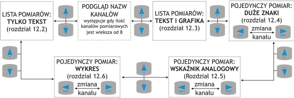
Rys.12. Schemat blokowy dostępnych trybów prezentacji danych pomiarowych Przykładowe zdjęcia ekranów rejestratora umieszczone poniżej mają charakter jedynie poglądowy, bazują na materiałach dotyczących podobnych urządzeń typu AR205/206.
