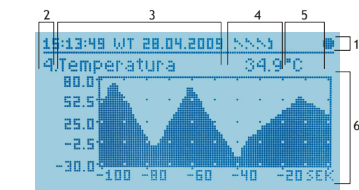
Rys.12.6. Wygląd ekranu pojedynczego pomiaru w trybie WYKRES
