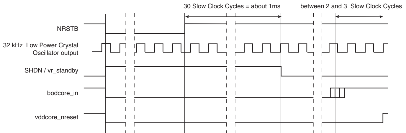
Figure 19-6. NRSTB Reset
