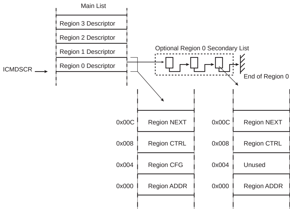
Figure 42-4. Region Descriptor
