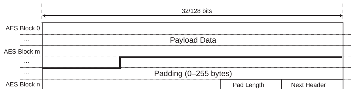
Figure 57-9. IPSEC Padding
