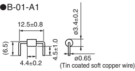
●B-01-A1
