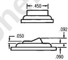
J50 Rocker Style w/Bezel
