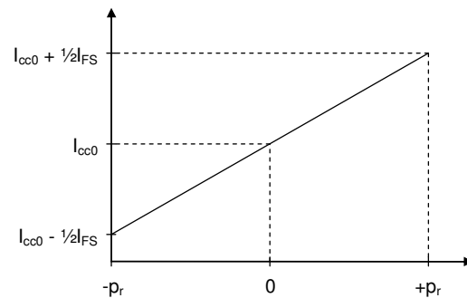
Symmetrical output (AUS)
