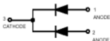
BAT54C (KL3)
