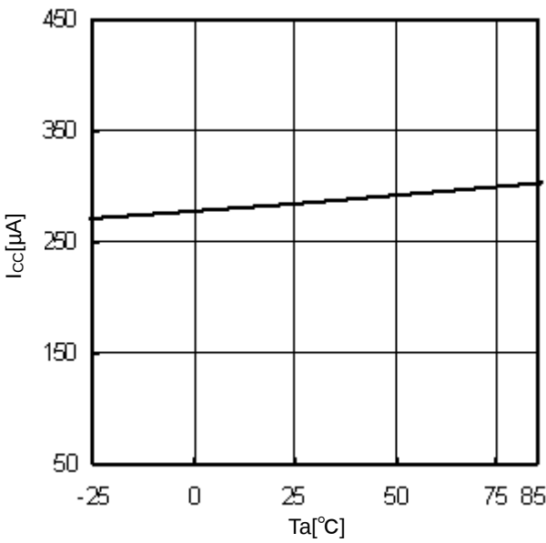
Fig.10 Ta- I_{CC}
