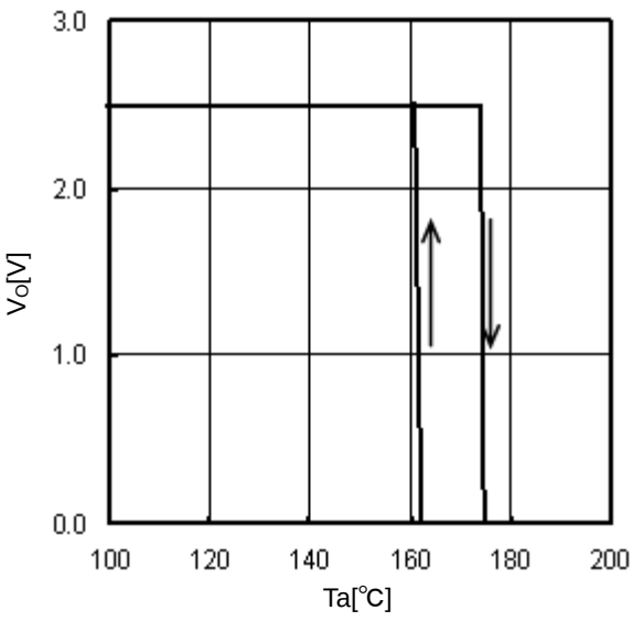
Fig.16 TSD ( I_O=0mA )
