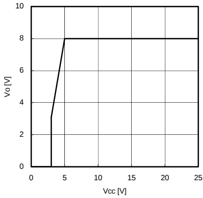
Fig.13 Vcc-Vo
