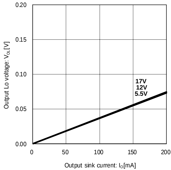
Fig. 20 Output Lo voltage ( T_a=25^\circ\text{C} )
