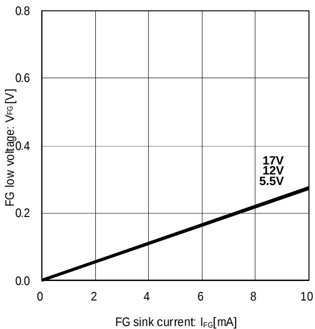
Fig. 9 FG low voltage (Ta=25°C)
