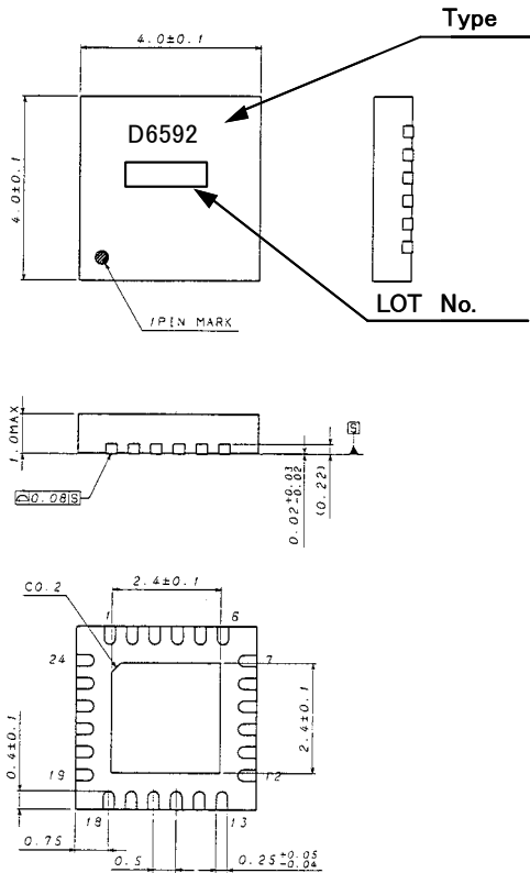
VQFN024V4040
