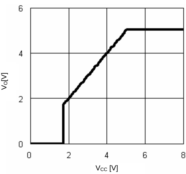
Fig.15 V_{CC}-V_O ( I_O=0mA )
