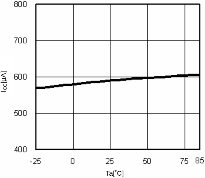
Fig.10 T_a-I_{CC}
