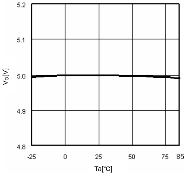
Fig.9 T_a-V_O ( I_o=0mA )
