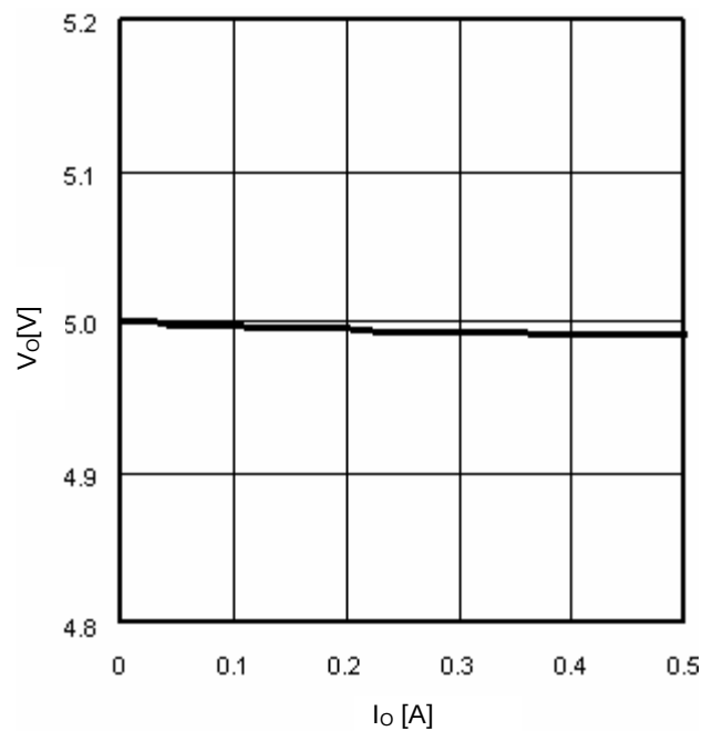
Fig.13 I_O - V_O
