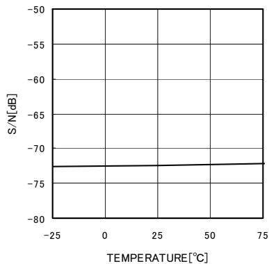
Fig.13 S/N
