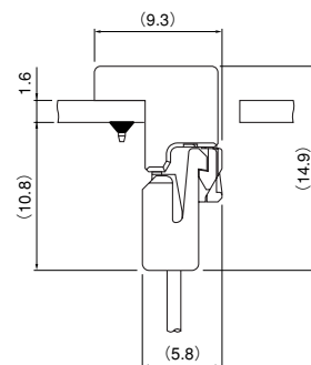
PAF Receptacle + PA bottom type header
