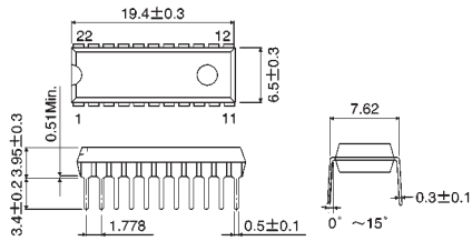
SDIP22
