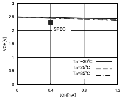
Fig.10 "H" output voltage VOH
