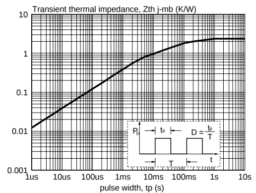
Fig.11. Transient thermal impedance; per diode; Z_{th\ j-mb} = f(t_p) .
