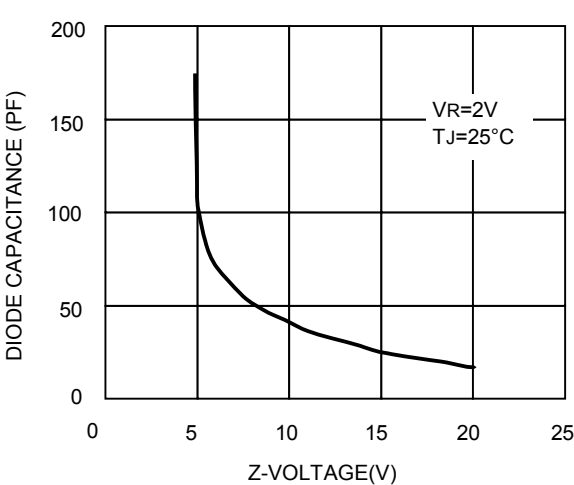
FIG.6 - DIODE CAPACITANCE VS.Z-VOLTAGE
