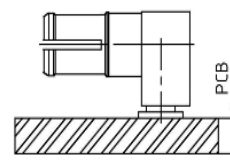
90° SMT
