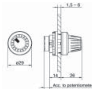
Potentiometer
