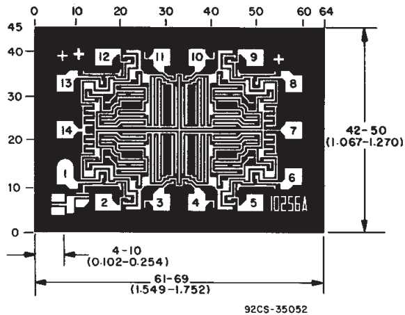
CD4011BH
