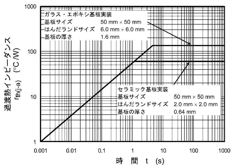
図 10.6 r_{th(j-a)} - t
