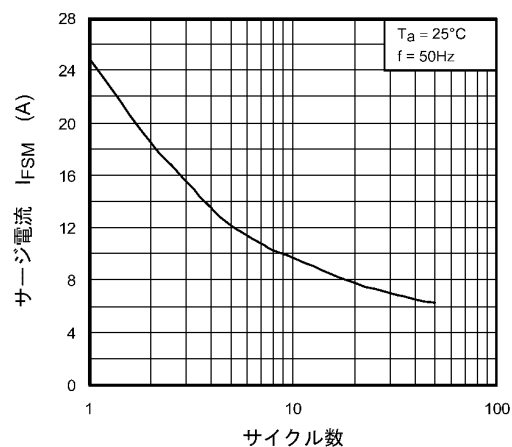
図 10.5 サージ電流
