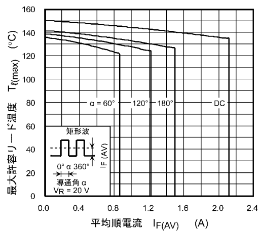
図 10.4 T_{t(max)} - I_{F(AV)}
