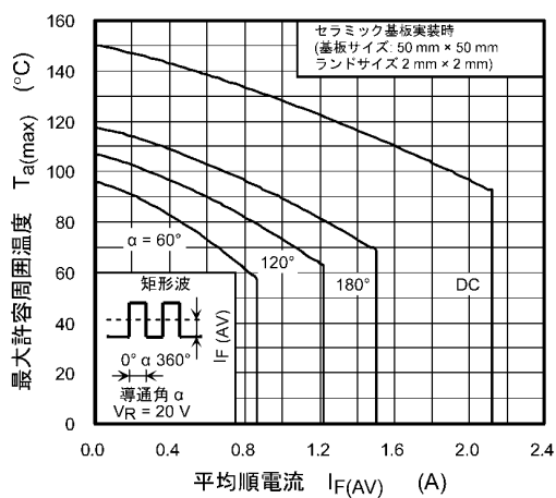
図 10.3 T_{a(max)} - I_{F(AV)}
