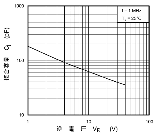
図 10.7 C_j - V_R
