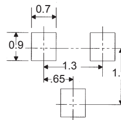
SOT-323
