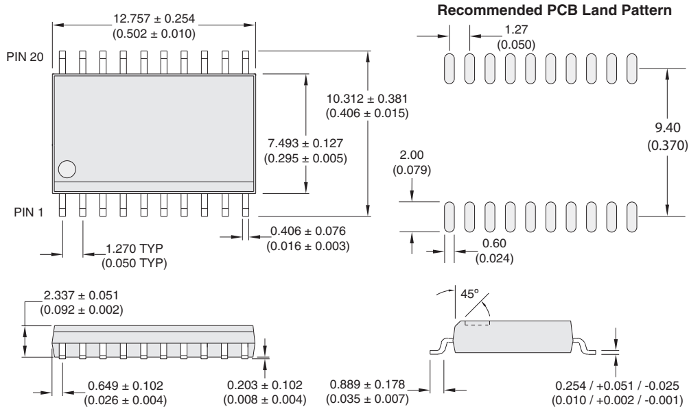
CPC7695Zx Package
