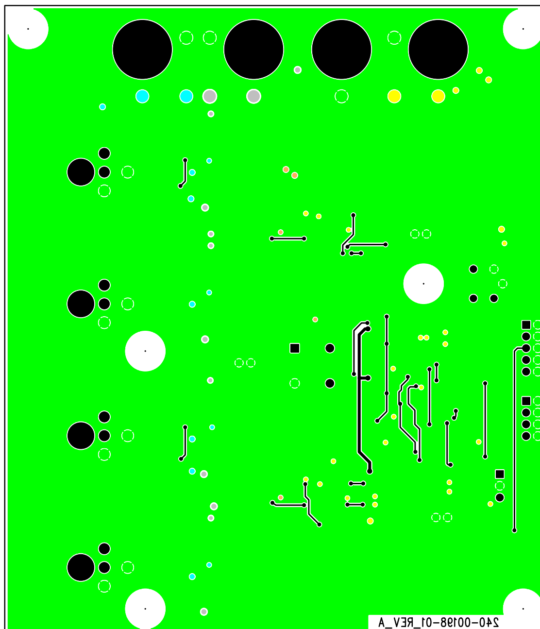
Figure 17. Bottom Layer
