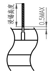
管脚处理示意图
