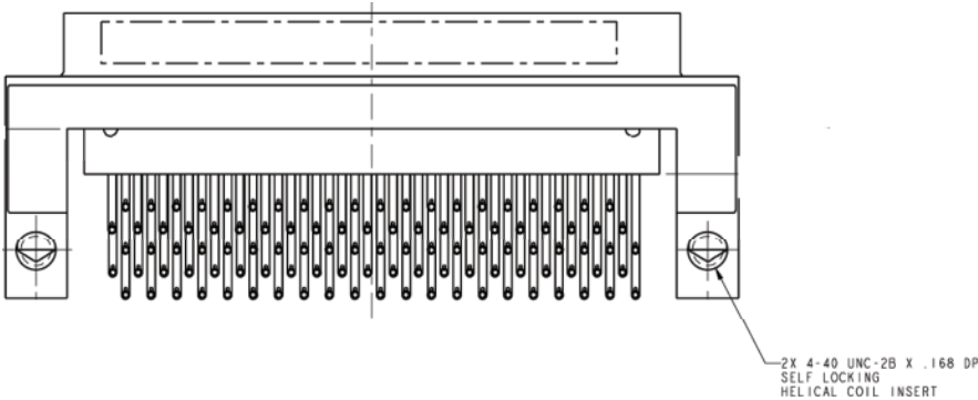
Receptacle - Socket
