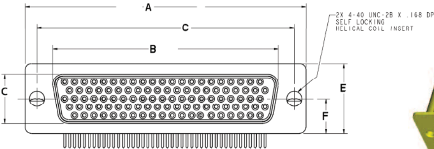
Receptacle - Socket
