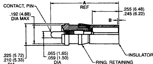
Receptacle
