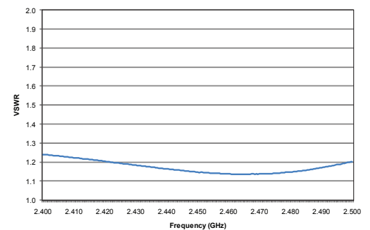
2400-2500 MHz
