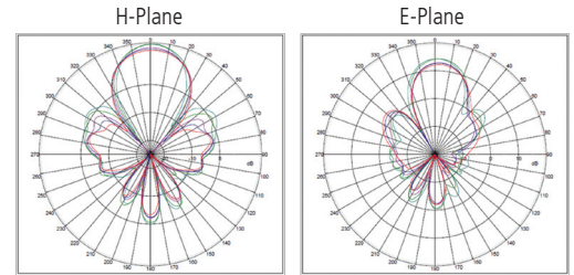
2400-2500 MHz
