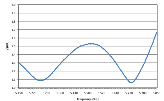
5150-5850 MHz
