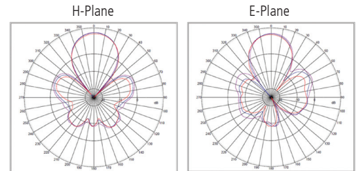
5150-5850 MHz
