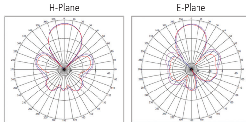
3300-3800 MHz
