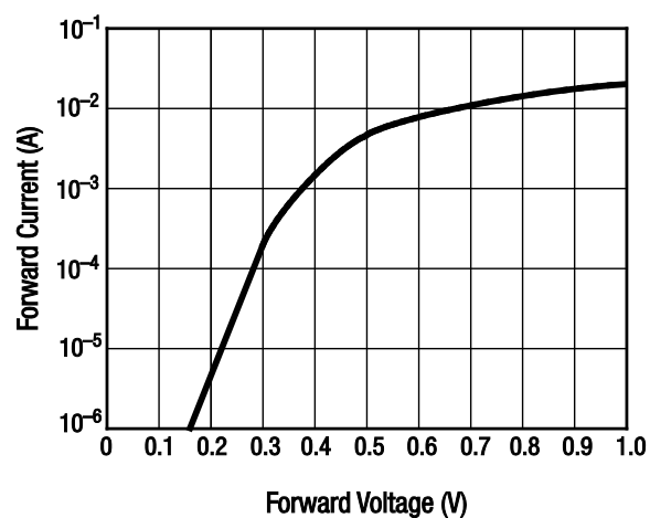
Figure 2. CDB7619-000
