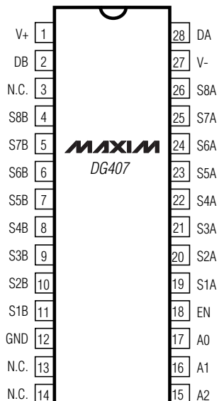
DIP/SO
