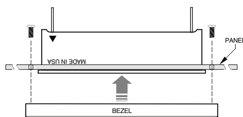
BEZEL INSTALLATION
