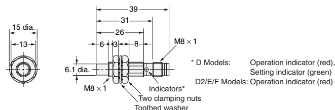
Diagram 29 E2E-X4MD□-M3G/E2E-X2ME□-M3/X2MF□-M3
