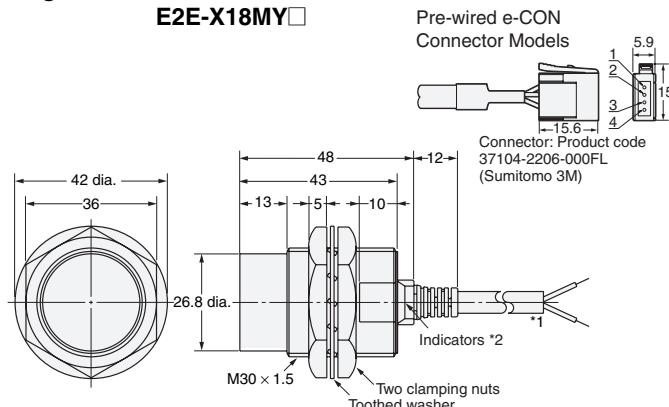
Diagram 17 E2E-X20MD□/E2E-X18ME□/F□ E2E-X18MY□
