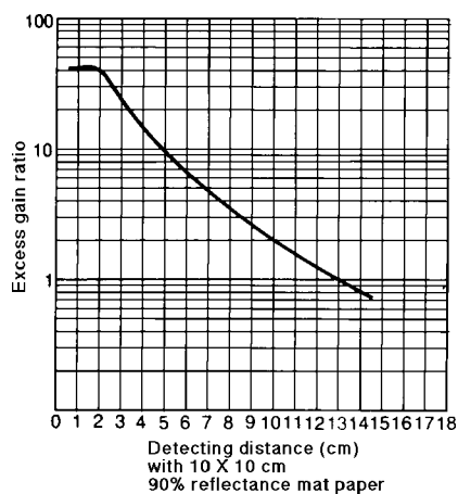
E3C-DS5W
