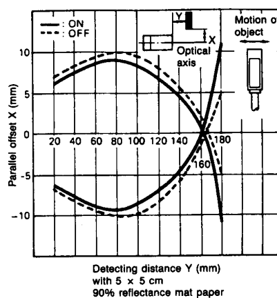
E3C-DS10 (Example 2)
