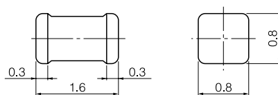
Type RE, PE (1.6×0.8×0.8)
