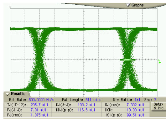
70m CAT5e - RX only
