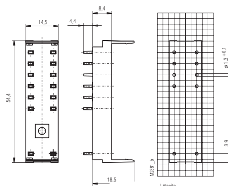
Lötseite
