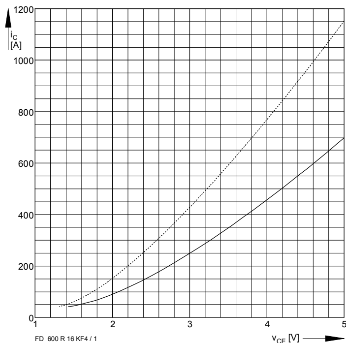
Bild / Fig. 1 Kollektor-Emitter-Spannung im Sättigungsbereich (typisch) / Collector-emitter-voltage in saturation region (typical) V_{GE} = 15 \text{ V} ..... t_{vj} = 25^\circ\text{C} ——— t_{vj} = 125^\circ\text{C}
