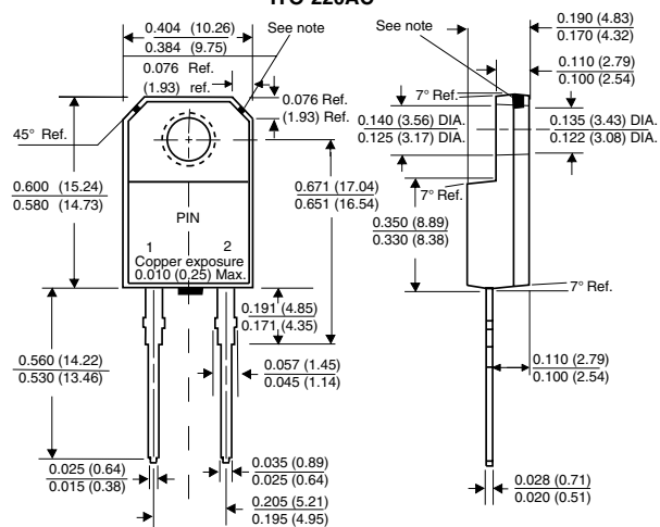
ITO-220AC
