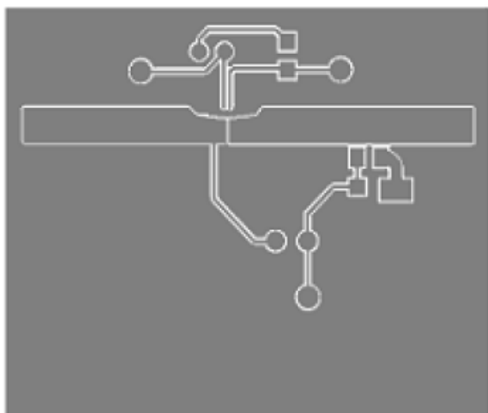
Figure 29. Top Layer
