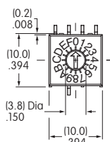
Hexadecimal
