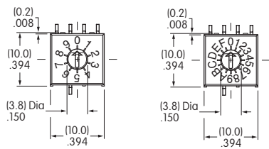
Decimal
