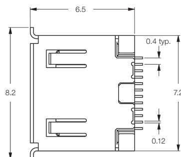
Receptacle
