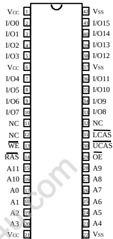
42 SOJ
