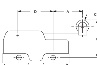
FIG. 1 Lever Roller
