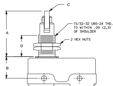
FIG. 6 Perpendicular Roller Plunger
