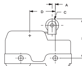
FIG. 2 Lever Roller
