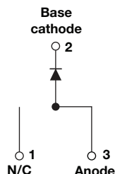
TO-263AB (D²PAK)
