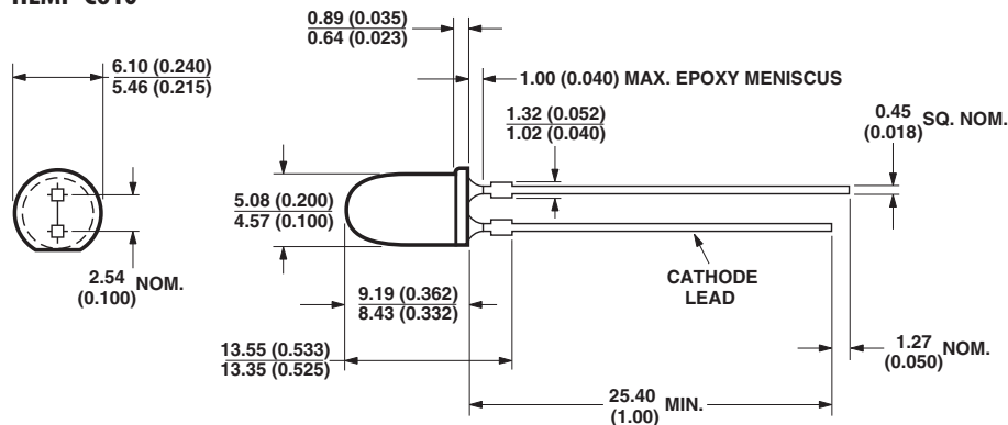
HLMP-C610
