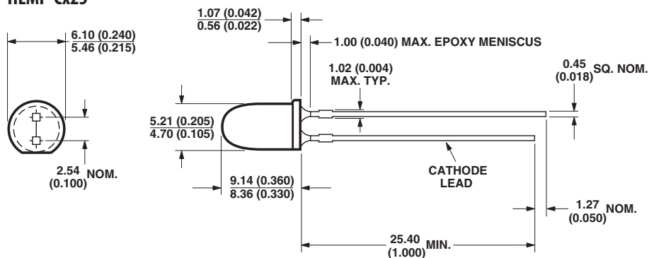
HLMP-Cx25
