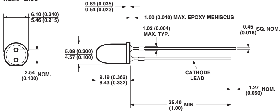
HLMP-Cx08
