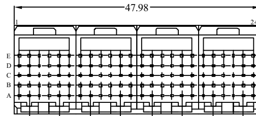
4 Module 89055-113LF
