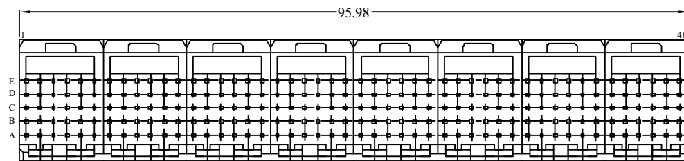
8 Module 89055-114LF
