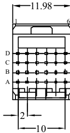
1 Module 70203-111LF
