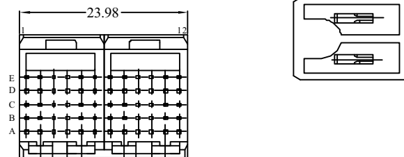
2 Module 89055-112LF
