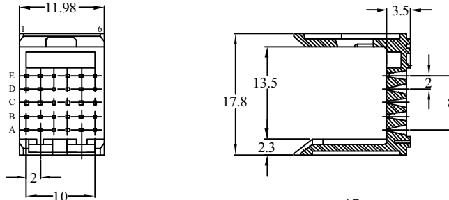
1 Module 89055-111LF
