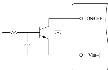
Fig. 15 Opto Coupler Enable Circuit
