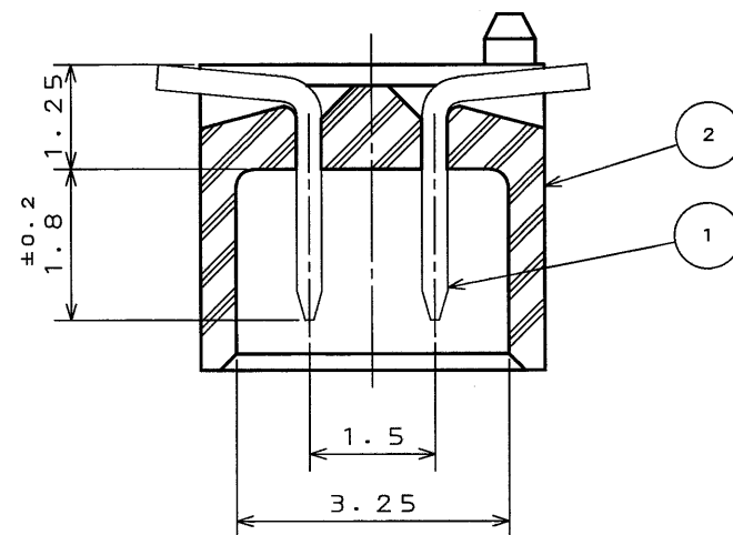
断面 A-A (尺度 10:1)
